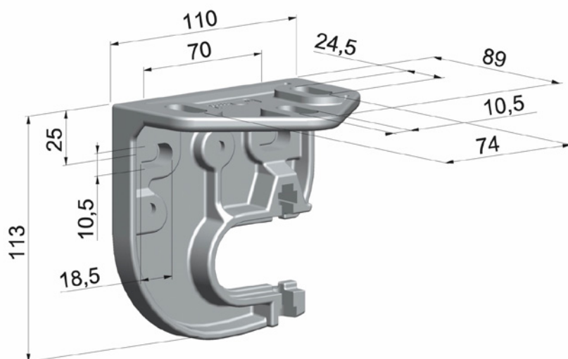
Sistema de Fijación del Perfil Frontal al Piso.
